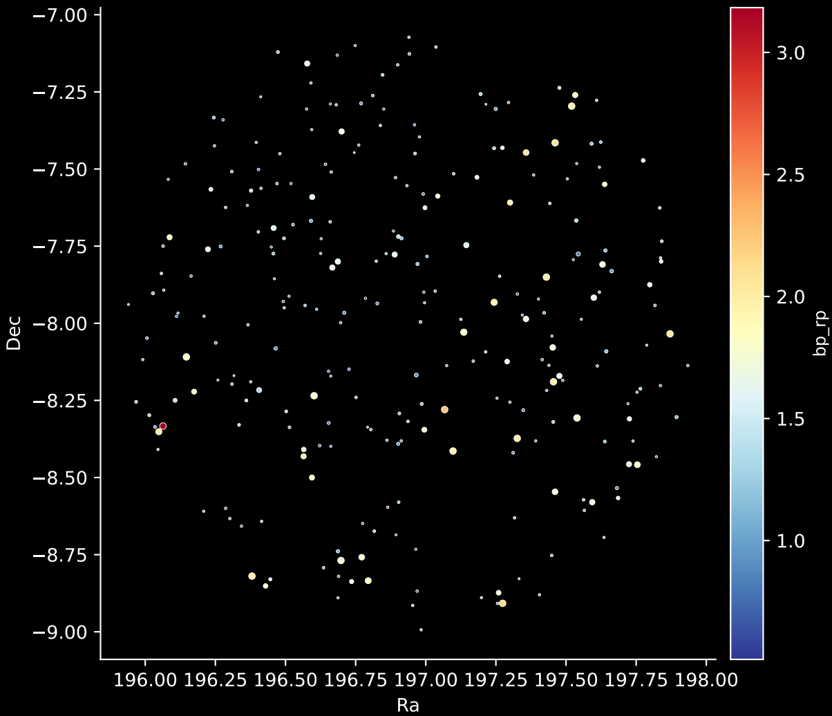
GALAH DR4 Field: [8958] Stars: 267
