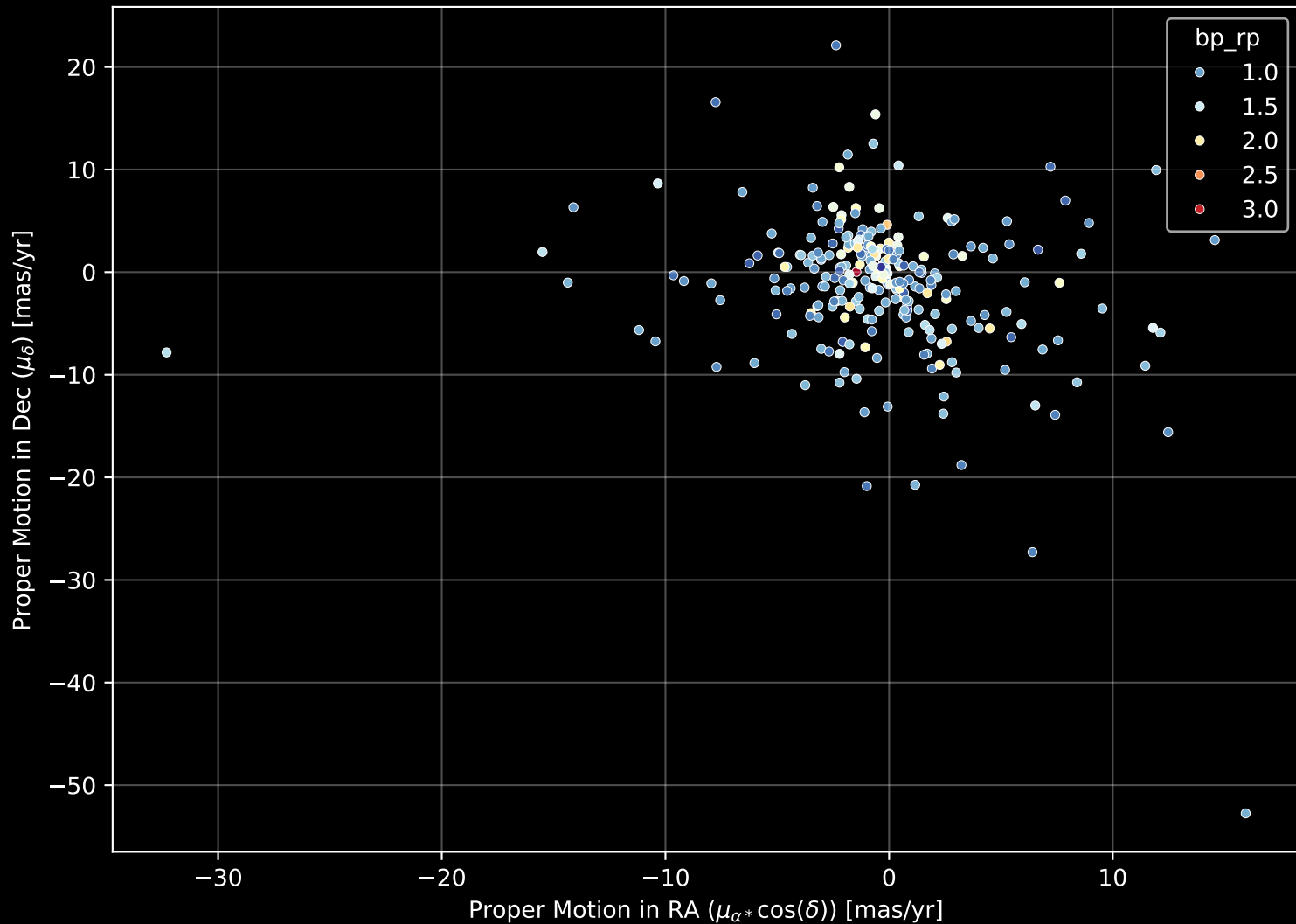
GALAH DR4 Field: [8958] Proper Motion Diagram (n= 267)
