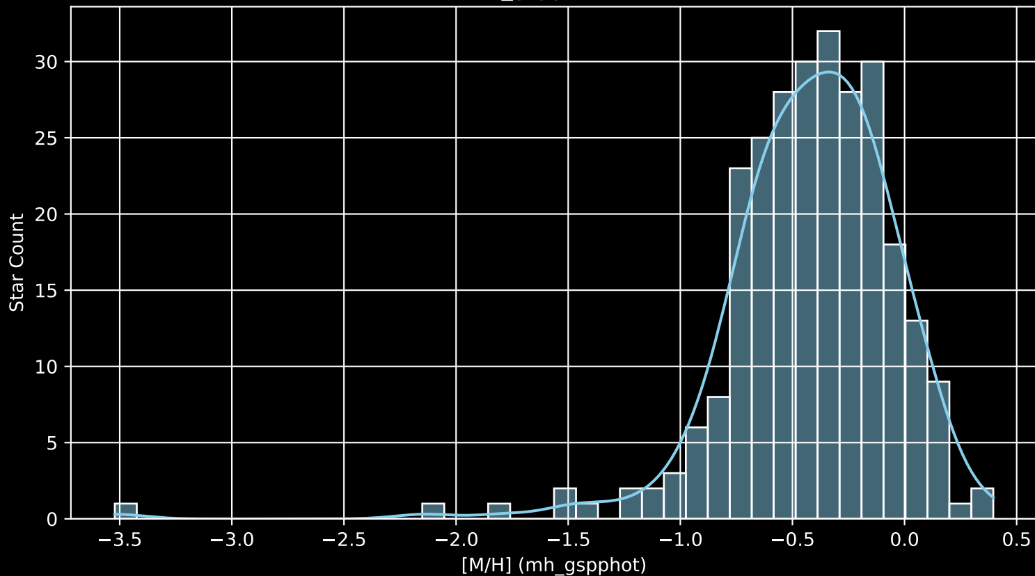
GALAH DR4 Field: [8958] [M/H] (mh_gspphot) (n= 266)
