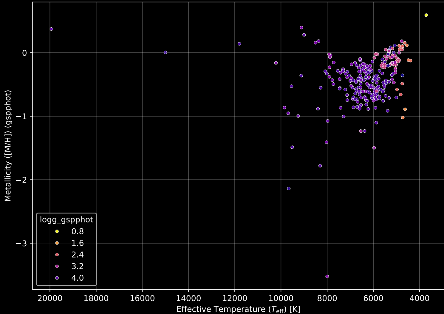
GALAH DR4 Field: [8958] Stellar Population Parameters (n= 267)
