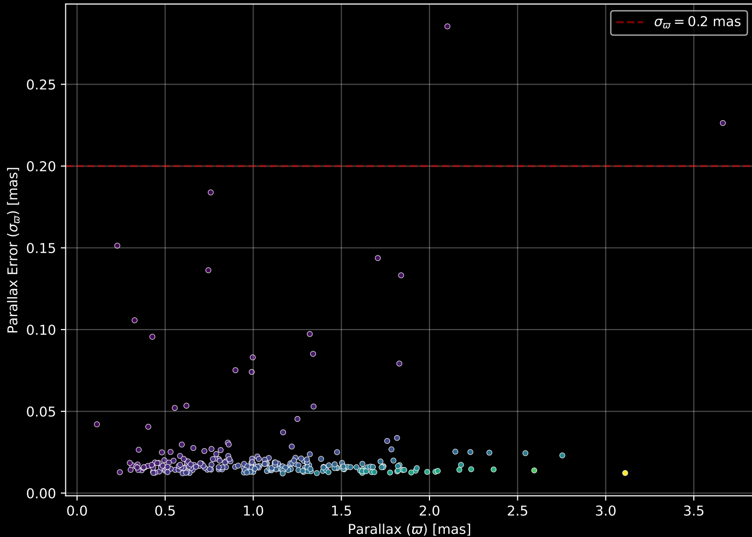
GALAH DR4 Field: [8958] Parallax Quality (n= 267)
